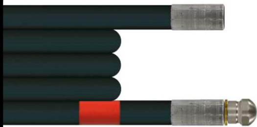
Geassembleerde flexibele slang 1SN
