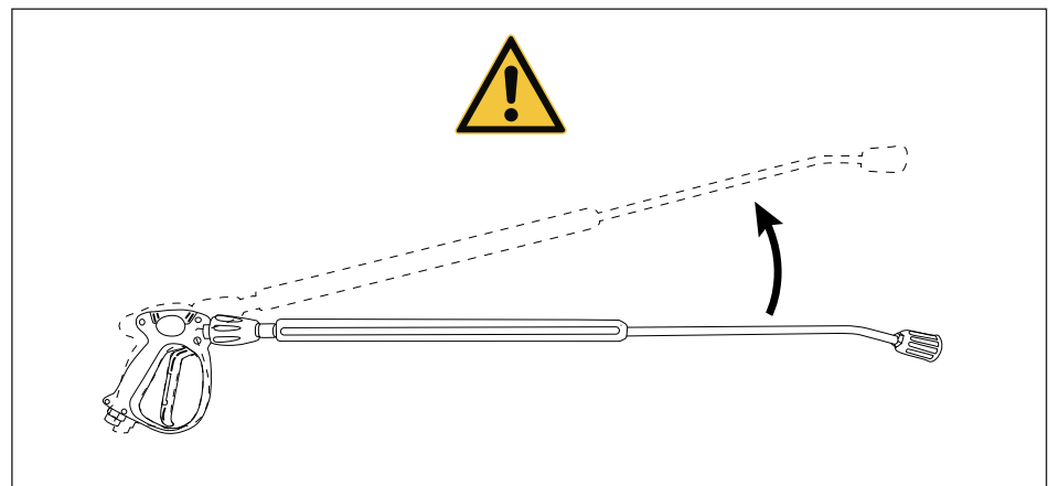
Abb. 6 - 7 Rückstoßkraft beim Einschalten der Abschalt pistole
